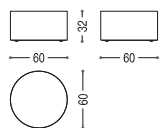
ECO 1 – CM. Ø 60 - H.32
