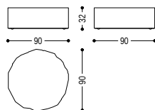
ECO 2 – CM. Ø 90 - H.32
